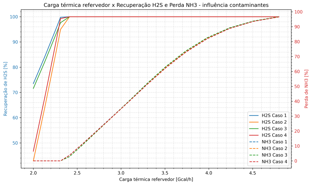
Figura 3: Carga térmica x recuperação de H_2S e perda de NH_3
