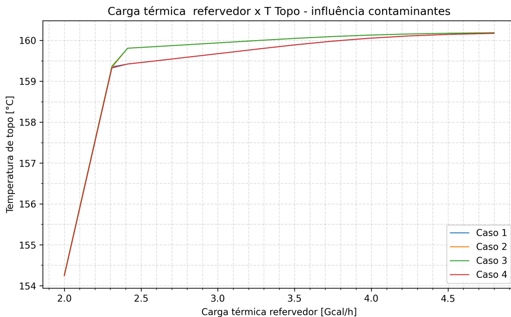
Figura 4: Carga térmica x Temperatura do topo da coluna
